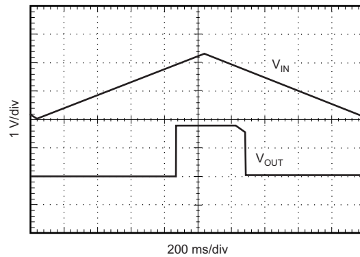
I OUT = 200 mA
